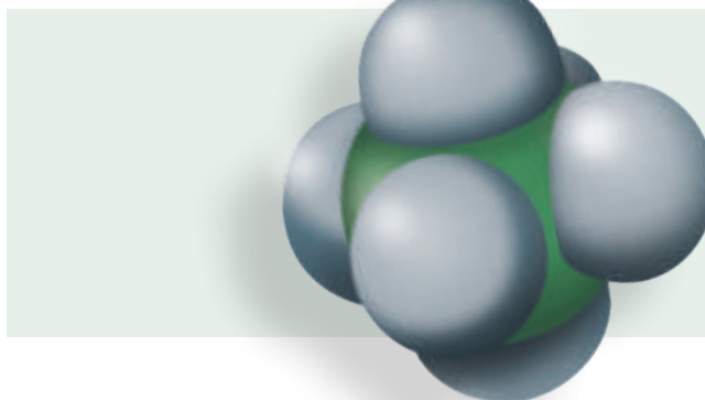
Модель молекулы гексафторида серы (один атом серы соединен с шестью атомами фтора)
